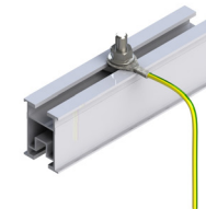
Befestigung des Erdungdrahts mittels Hammerkopfschraube
