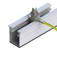
Befestigung des Erdungdrahts mittels Hammerkopfschraube
