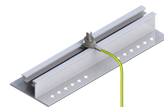
Befestigung des Erdungdrahts mittels Hammerkopfschraube
